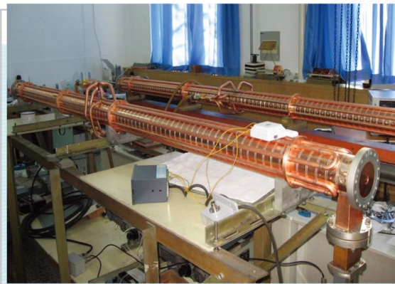
■ 加速管
